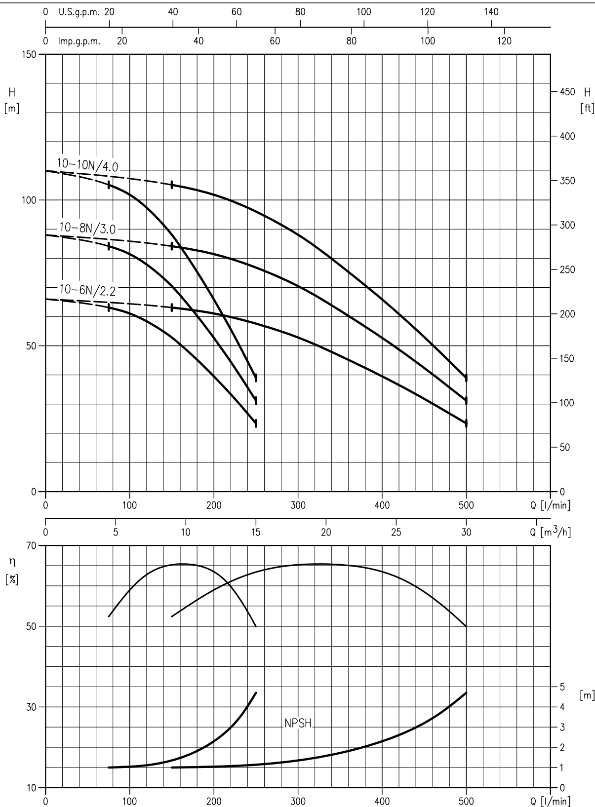
COURBES DE PERFORMANCE série 2GPE EVMG 10 E -drive (selon ISO 9906 annexe A)
