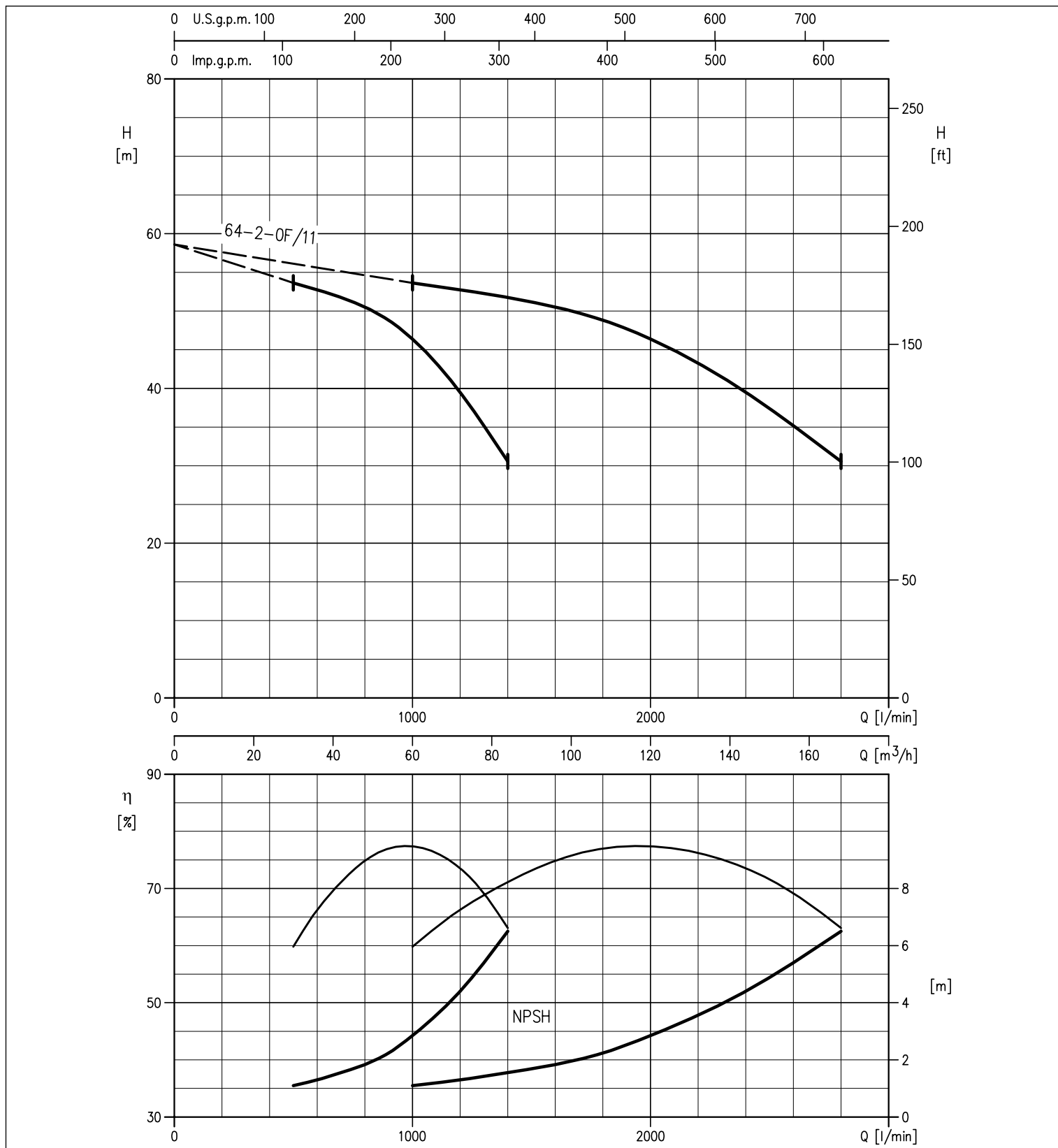
COURBES DE PERFORMANCE série 2GPE EVMG 64 E-drive (selon ISO 9906 annexe A)
