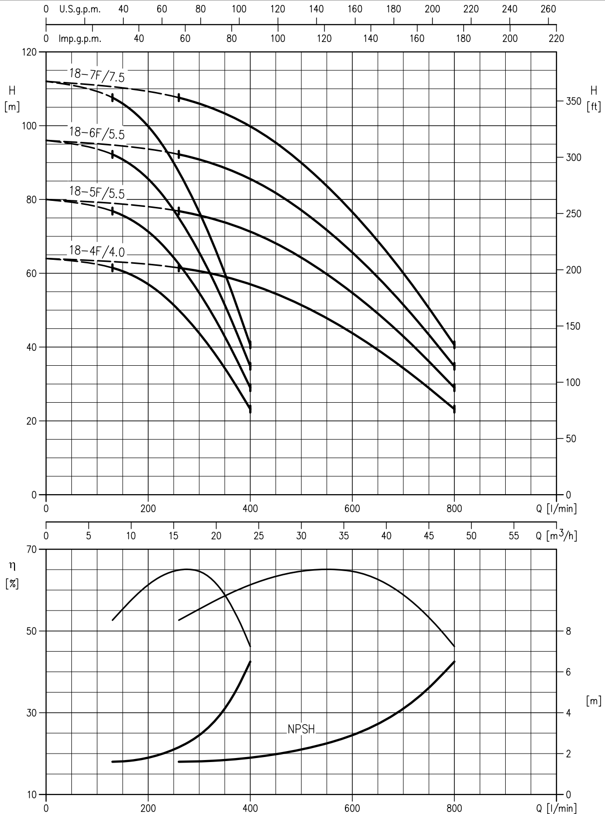
COURBES DE PERFORMANCE série 2GPE EVMG 18 E-drive (selon ISO 9906 annexe A)
