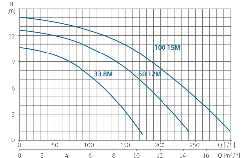
Courbes de fonctionnement à 2900 rpm
