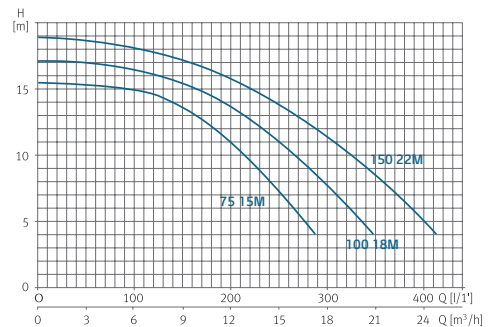
Courbes de fonctionnement à 2900 rpm
