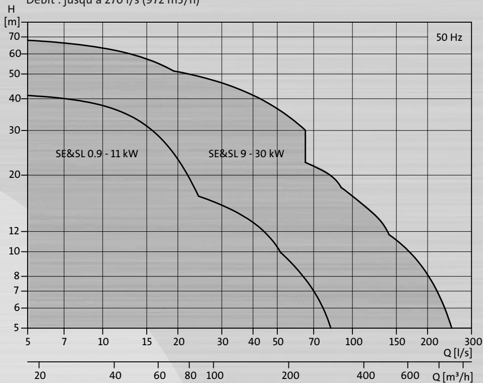
Courbe de performance des pompes SE et SL combinées
