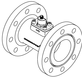
Fig. 26 VFI sensor
