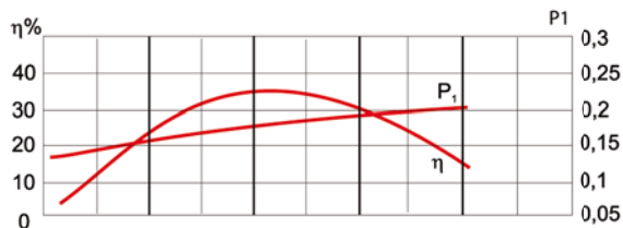
Courbes hydrauliques
