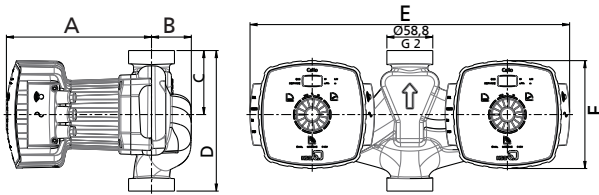
Pompe à orifices filetés
