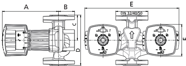
Pompe à brides
