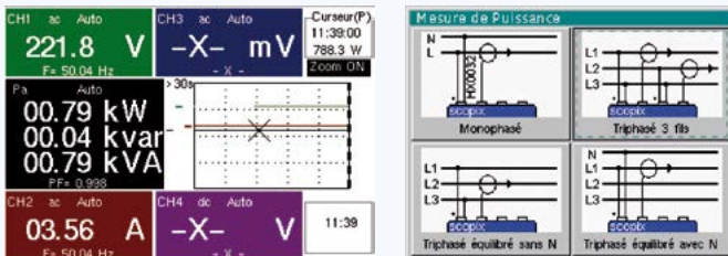
Affichage des puissances apparente, active, réactive et du PF
