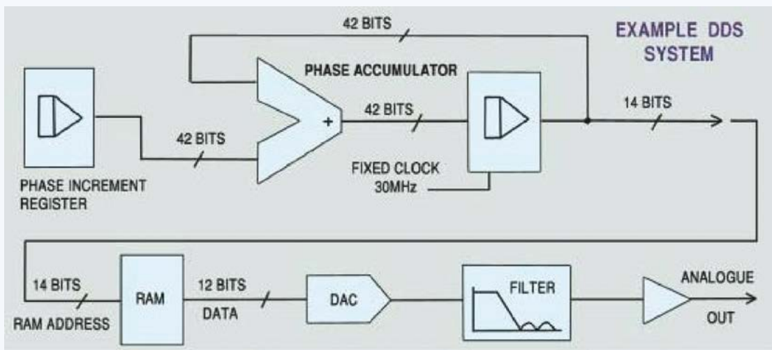
Architecture d'un générateur de Fonctions à synthèse numérique Directe (DDS)
