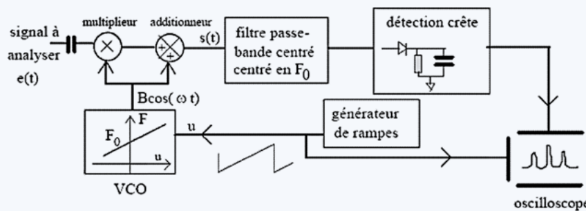
Synoptique d'un analyseur de spectre hétérodyne
