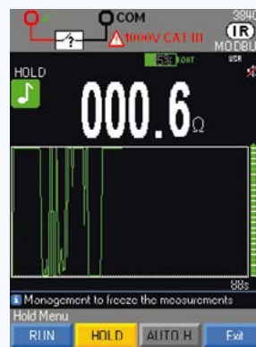
Écran graphique couleur
