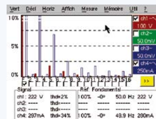
Le zoom vertical (bouton face avant) permet de pouvoir régler la dynamique en fonction du besoin (0-100 %, 0-50 %, 0-25 % ou 0 - 10 %)
