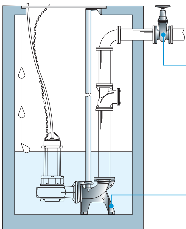
Dispositif d'accouplement de fond à refoulement vertical avec système de décrochage BREVETÉ Dispositivo de acoplamiento de fondo con alimentación vertical y sistema de desenganche PATENTADO
