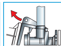
Dispositif d'accouplement de fond à refoulement vertical avec système de décrochage BREVETÉ Dispositivo de acoplamiento de fondo con alimentación vertical y sistema de desenganche PATENTADO
