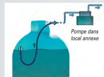
Installation avec pompe de surface
