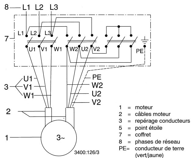
Branchement d'un moteur à couplage étoile-triangle et avec 2 câbles pour démarrage étoile-triangle.
